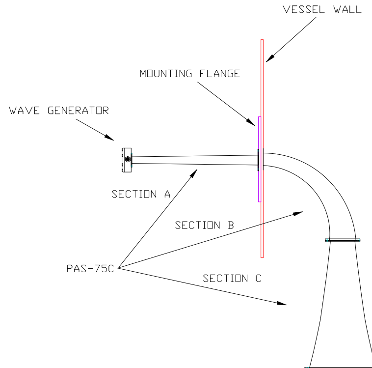
DRAWING N° 75C-SD2
