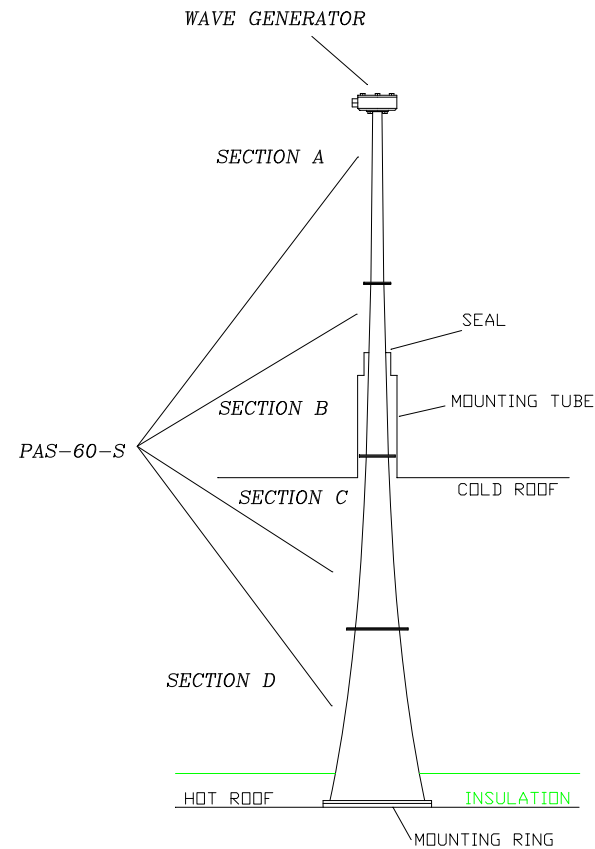
DRAWING N° 060-S-SD6
