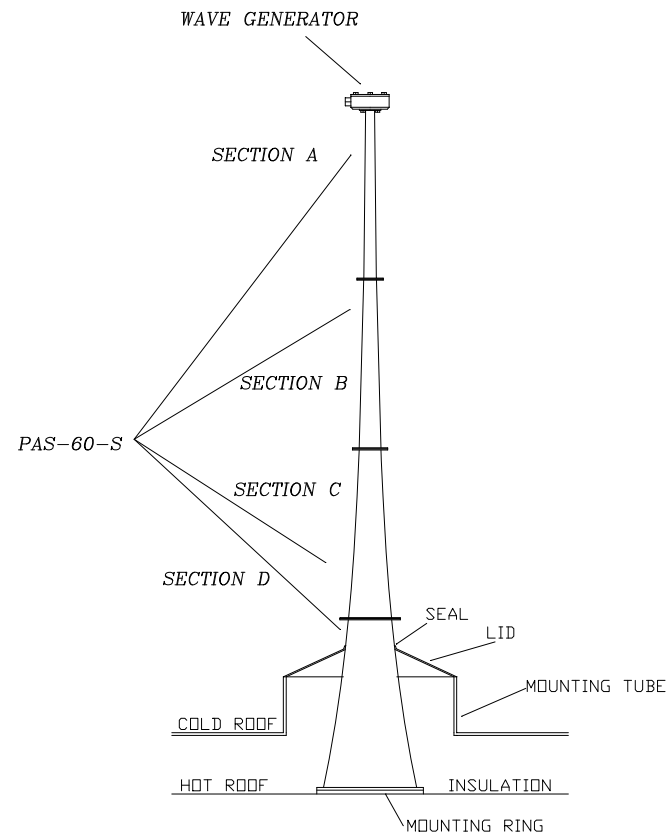
DRAWING N° 060-S-SD5
