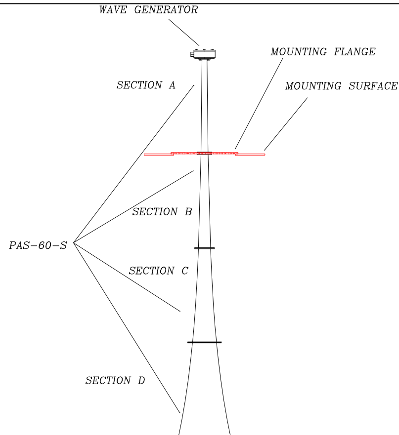
DRAWING N° 060-S-SD4
