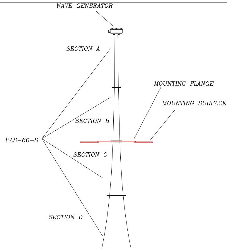
DRAWING N° 060- S-SD3
