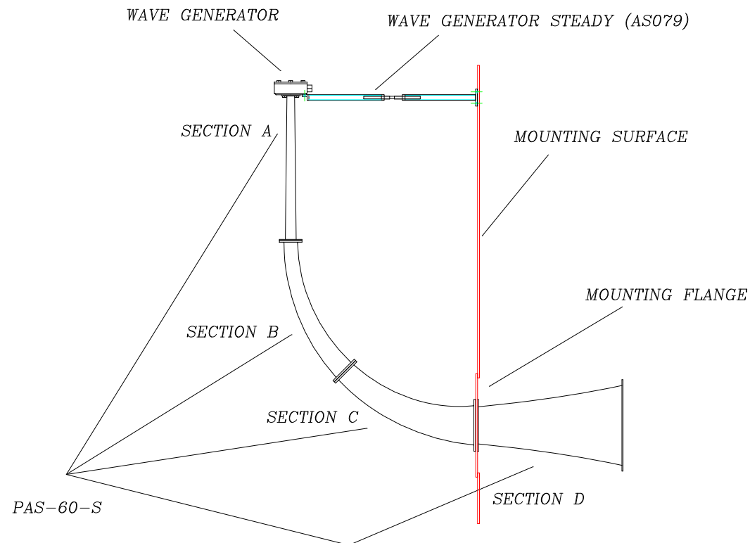
DRAWING N° 060-C-SD2
