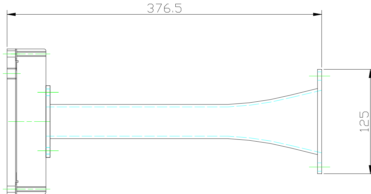
Drawing N° - AS020 Audiosonic™ Range – Model PAS 420
